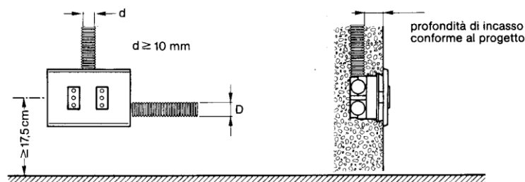
Figura 30.1 Criteri di installazione degli impianti incassati e similari
