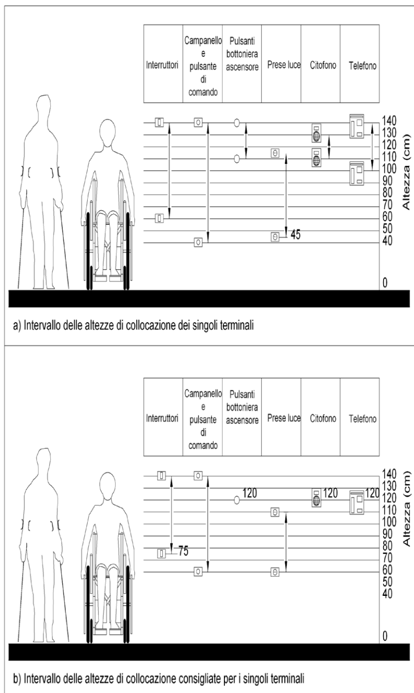
Figura 30.2 Altezze consigliate per i terminali degli impianti elettrici e telefonici
